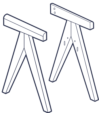
■ Leg × 2
